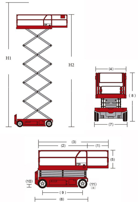
Diagrama de dimensiones del equipo
